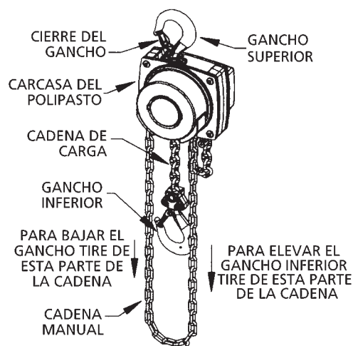
Figura 2 - Piezas principales del polipasto Hurricane
