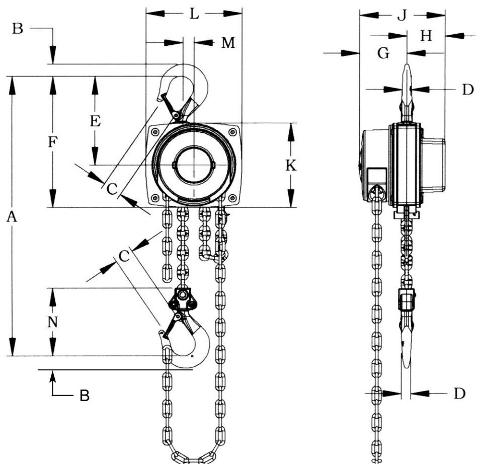
Figure 1 - Spécifications
