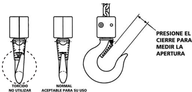
Figura 3 – Inspección del gancho
