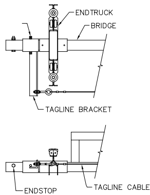
Diagram 9A. Tagline on steel bridge.
