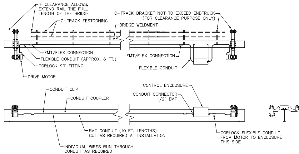
Diagram 9A. Bridge conduit wiring diagram.
