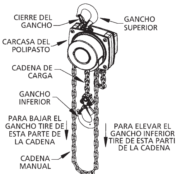
Figura 2 – Piezas principales del polipasto Hurricane 360
